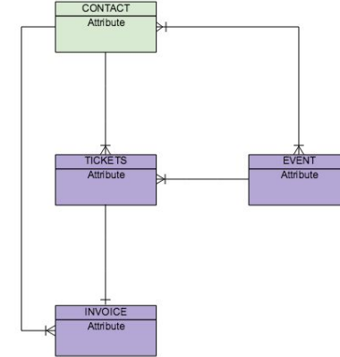
SFDC DATA MODEL
